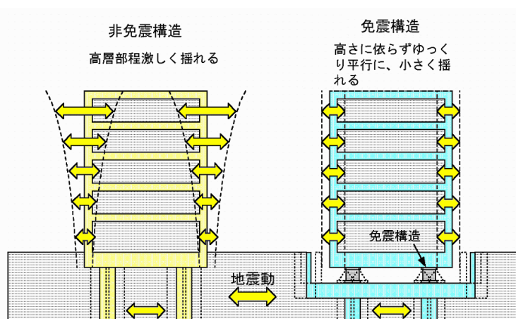
図5 非免震・免震構造の応答挙動の概念
